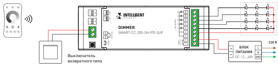
Рис. 5. Схема подключения диммера для управления DIM-нагрузкой
