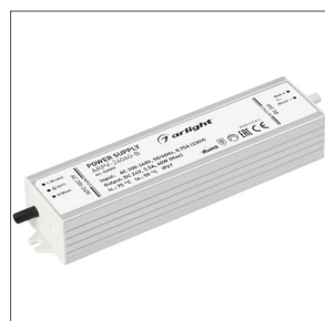
020005 | Блок питания ARPV-24060-B (24V, 2.5A, 60W)
