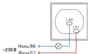
Рис. 1. Схема подключения
