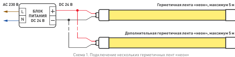
Схема 1. Подключение нескольких герметичных лент «неон»
