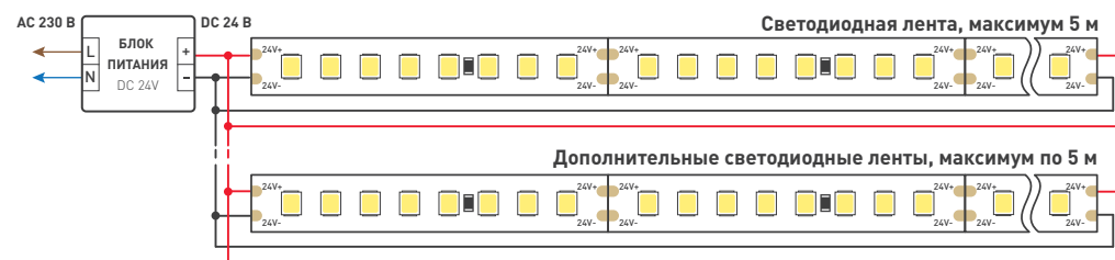
Рис. 2. Подключение нескольких светодиодных лент с двух сторон
