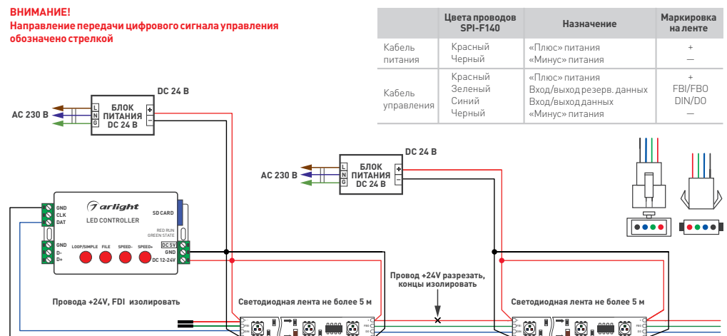
Схема 1. Подключение ленты с использованием SPI-контроллера с одним выходным портом и с использованием отдельных блоков питания.
