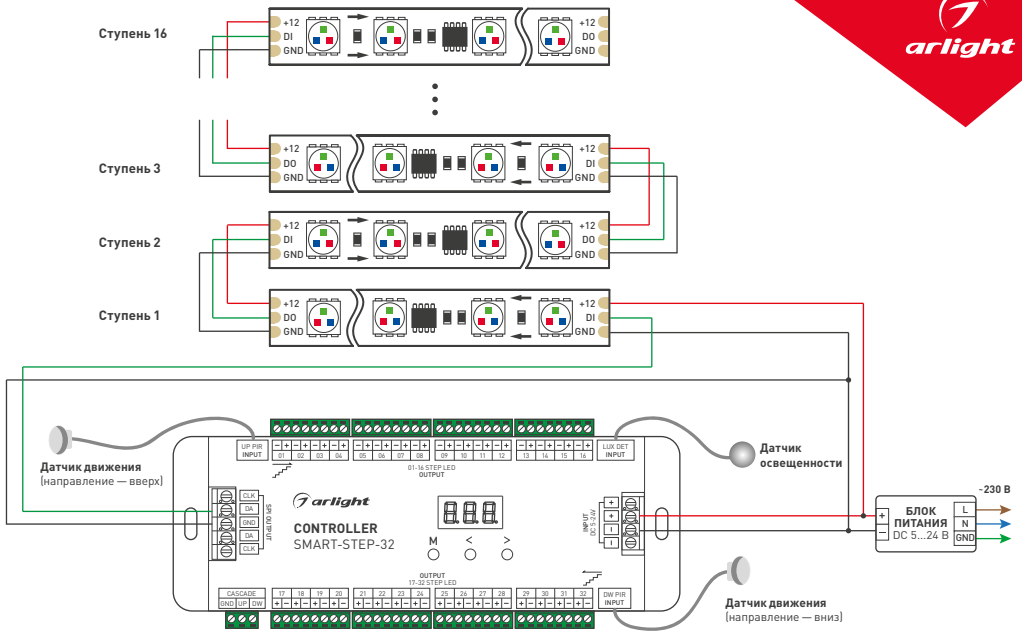
Рис. 3. Схема подключения контроллера в режиме управления светодиодной лентой SPI (ступени) Color_Step
